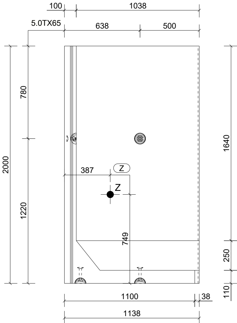
Aanzicht B Schaal: 1:20
