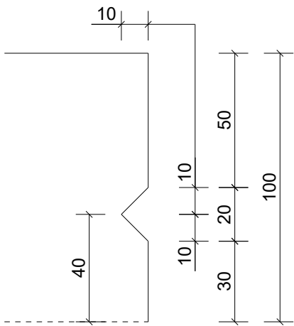
Detail A, 1:2
