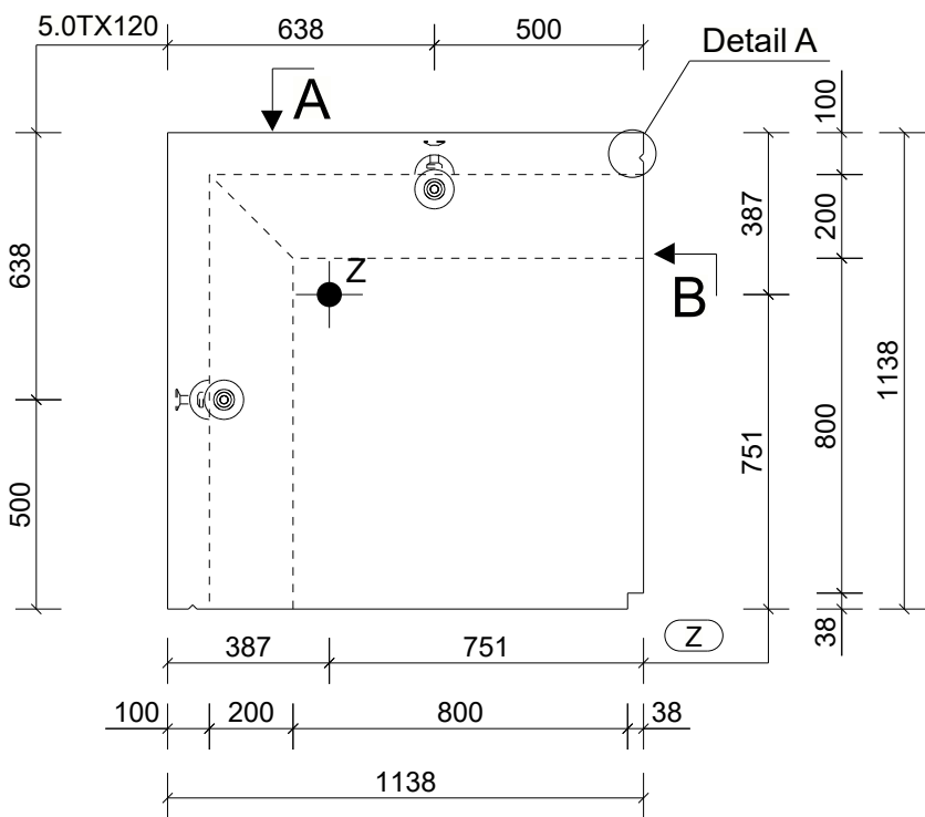
Aanzicht C Schaal: 1:20
