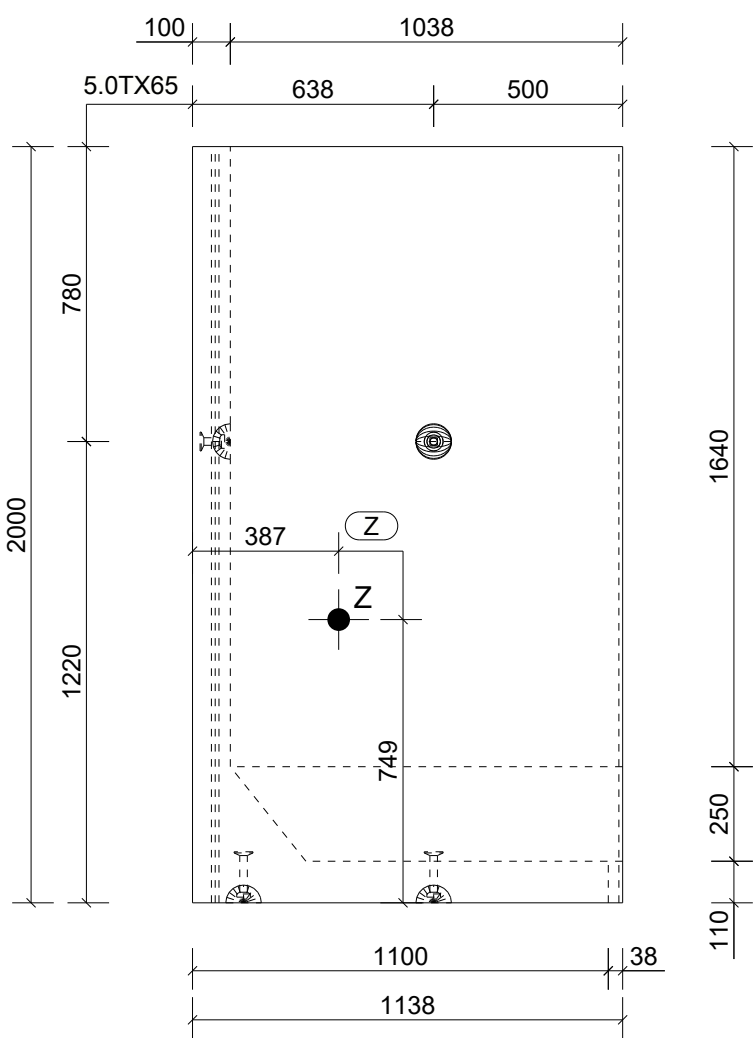
Aanzicht A Schaal: 1:20
