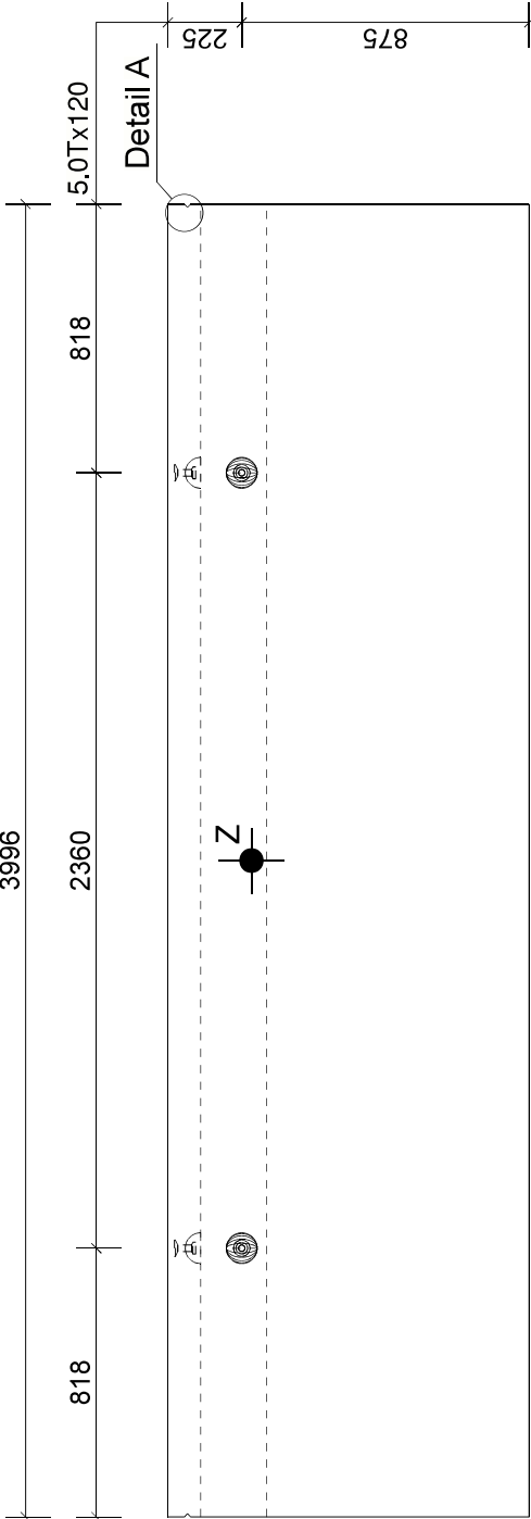
Aanzicht A
