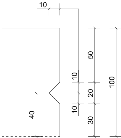
Detail A, 1:2
