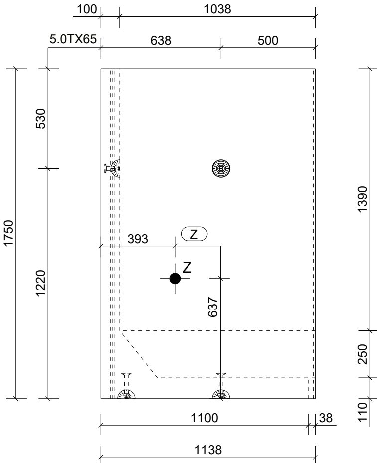
Aanzicht A Schaal: 1:20
