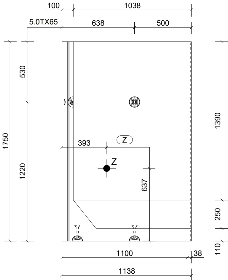
Aanzicht B Schaal: 1:20
