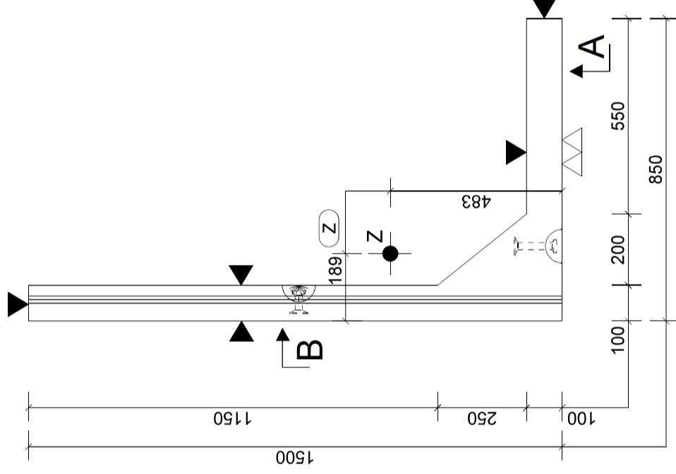
Doorsnede Schaal: 1:15
