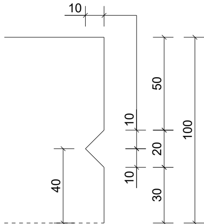
Detail A, 1:2
