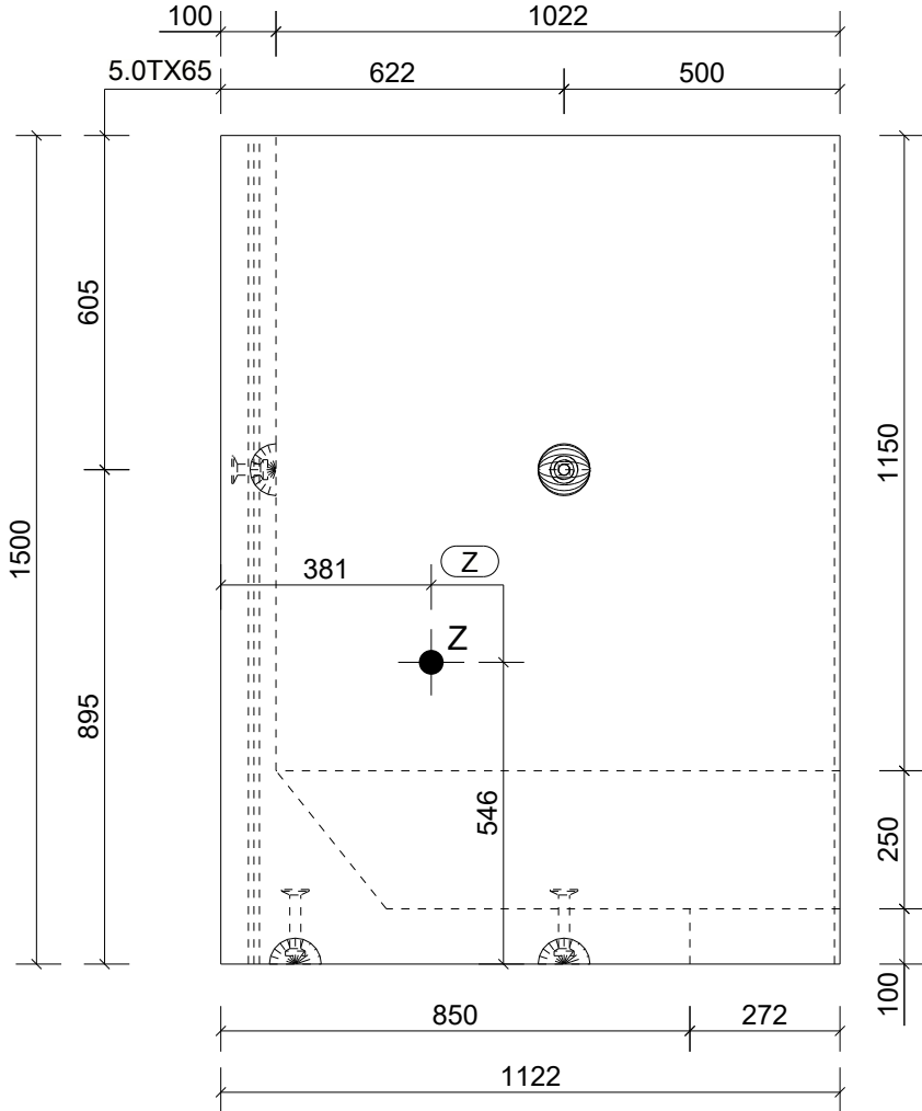
Aanzicht A Schaal: 1:15
