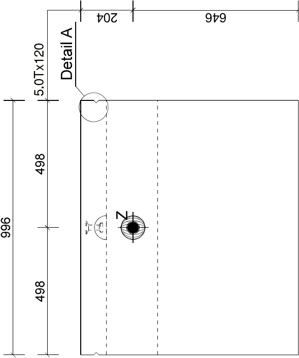
Aanzicht A Schaal: 1:15
