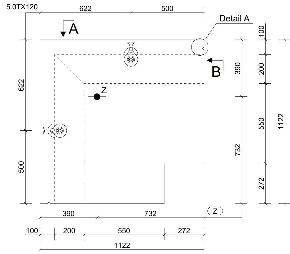
Aanzicht C Schaal: 1:15
