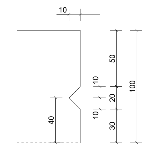
Detail A, 1:2
