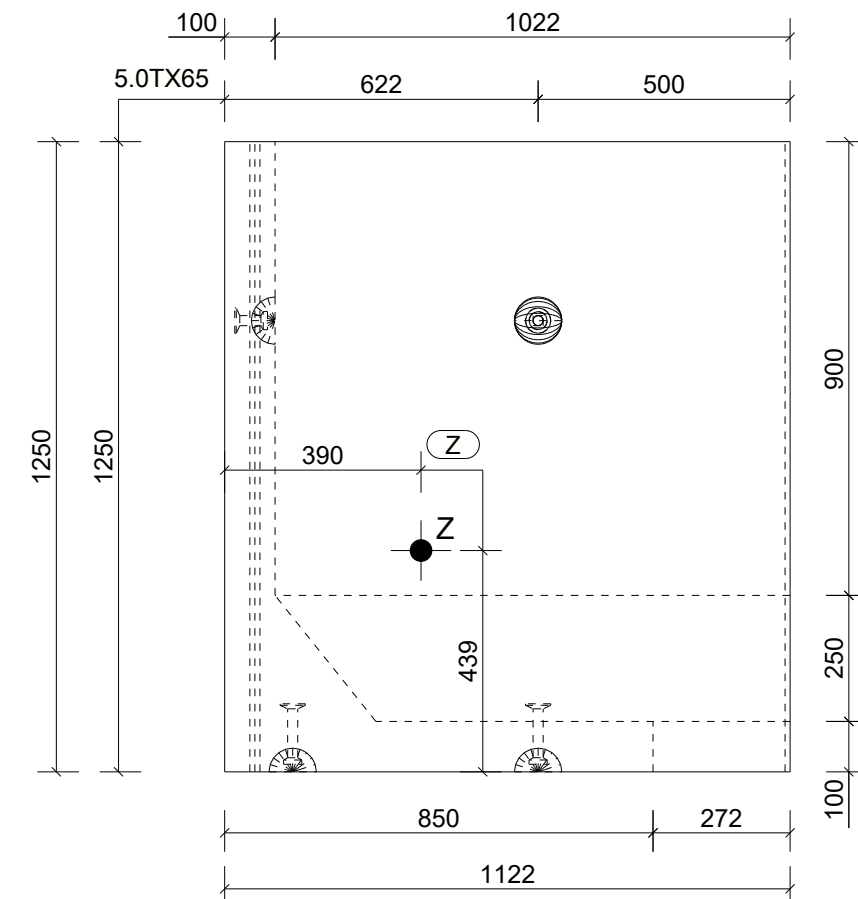
Aanzicht A Schaal: 1:15
