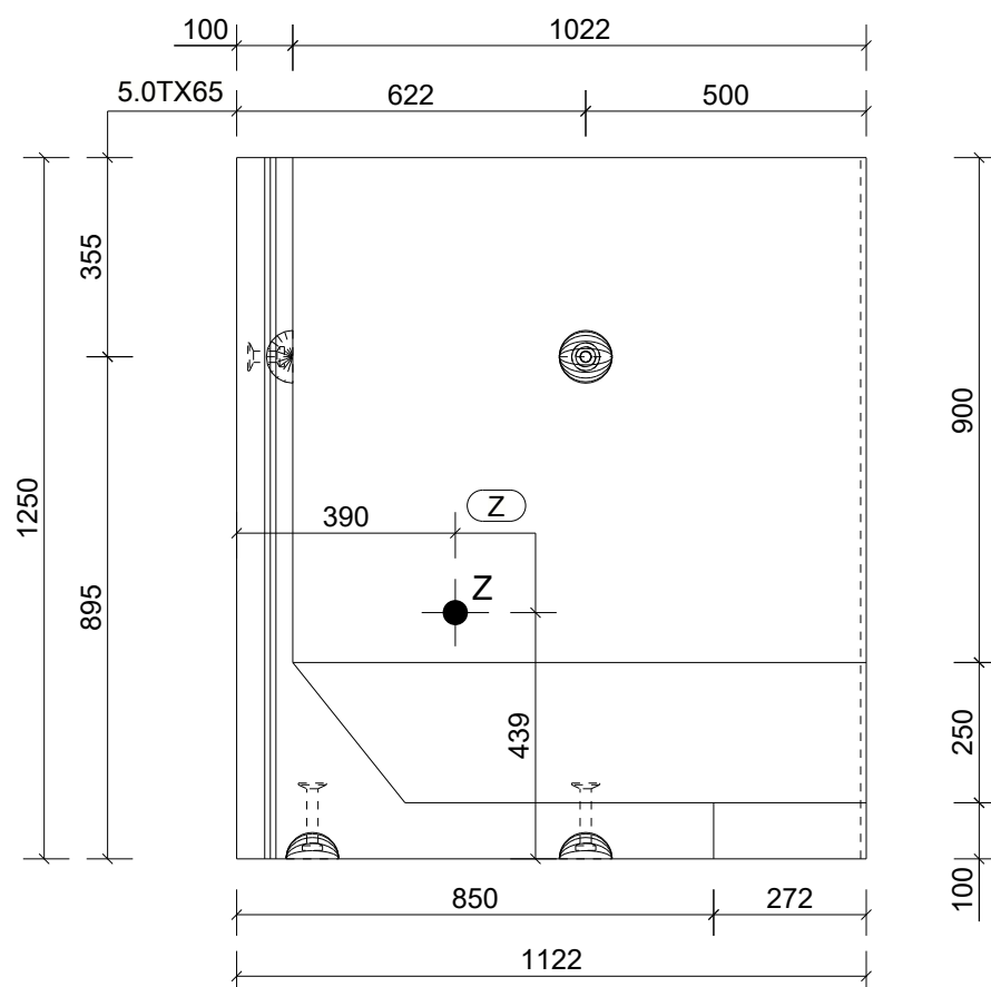
Aanzicht B Schaal: 1:15
