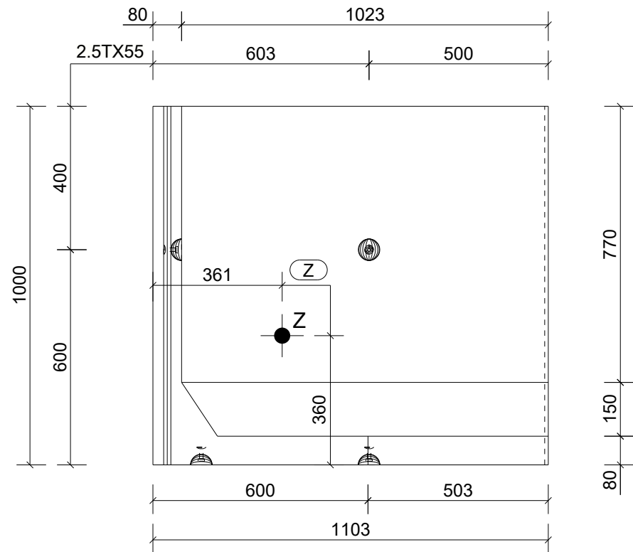
Aanzicht B Schaal: 1:15
