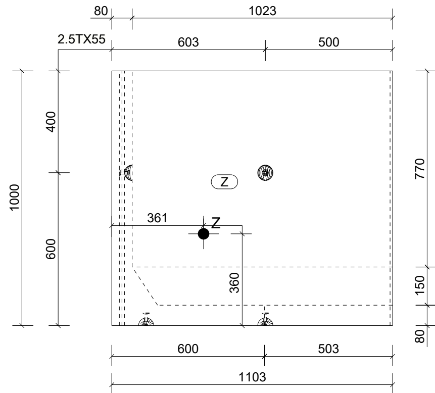
Aanzicht A Schaal: 1:15
