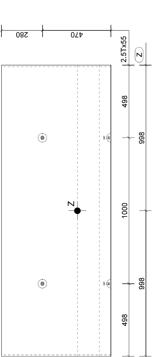
Aanzicht B Schaal: 1:15
