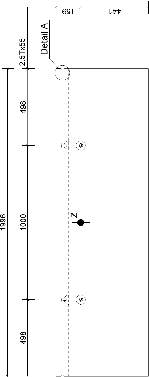
Aanzicht A Schaal: 1:15
