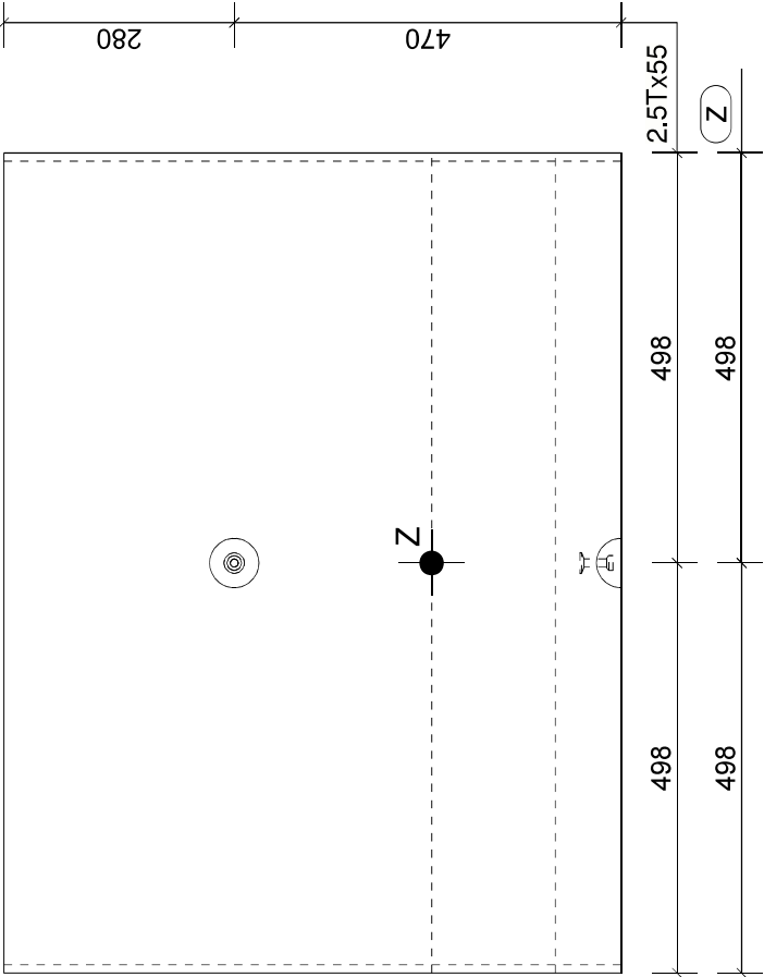
Aanzicht B Schaal: 1:10
