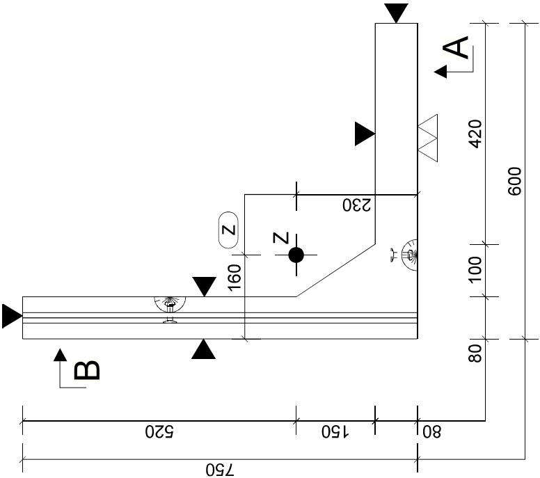
Doorsnede Schaal: 1:10
