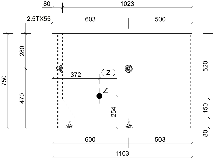
Aanzicht A Schaal: 1:15
