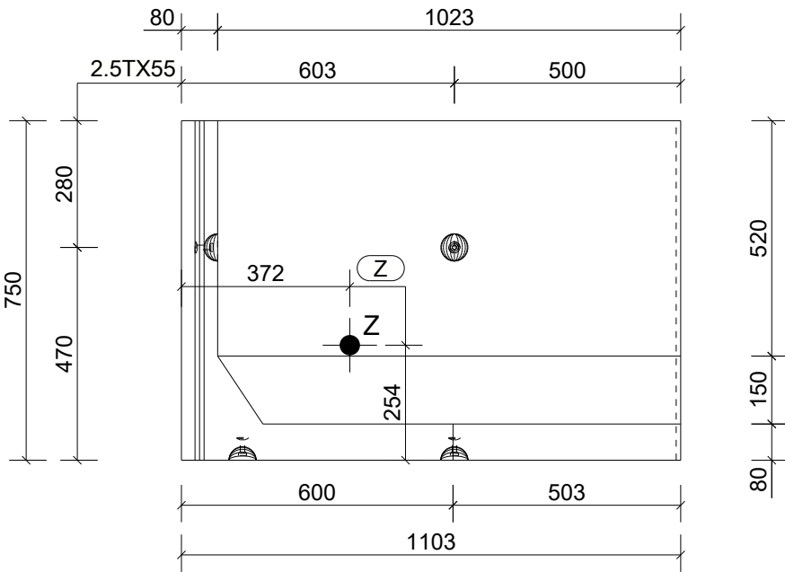
Aanzicht B Schaal: 1:15
