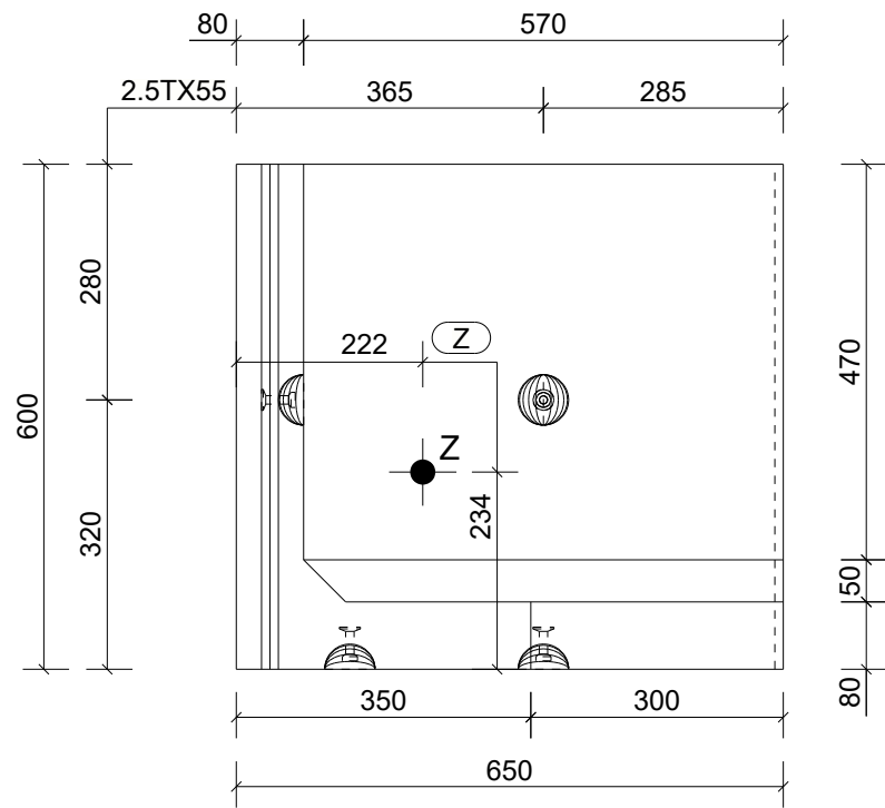
Aanzicht B Schaal: 1:10
