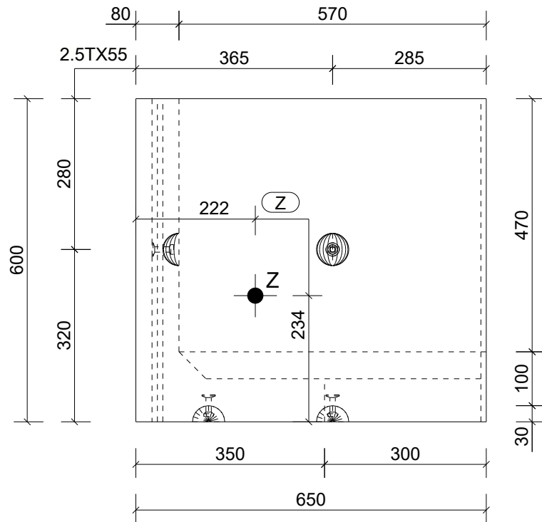
Aanzicht A Schaal: 1:10
