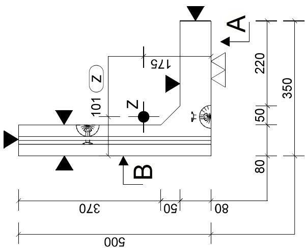
Doorsnede Schaal: 1:10
