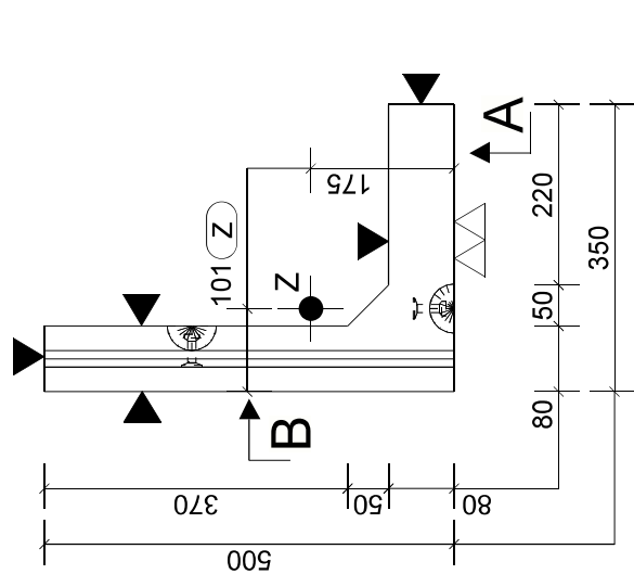
Doorsnede
