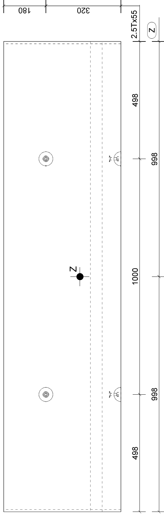
Aanzicht B
