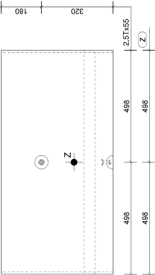
Aanzicht B Schaal: 1:10
