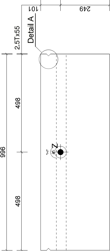
Aanzicht A Schaal: 1:10
