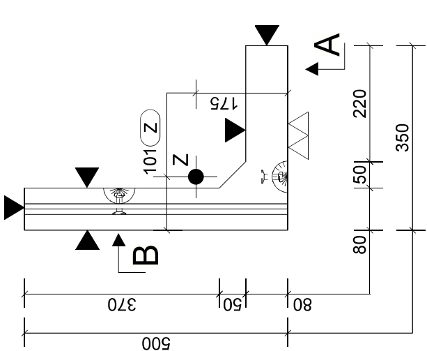
Doorsnede Schaal: 1:10
