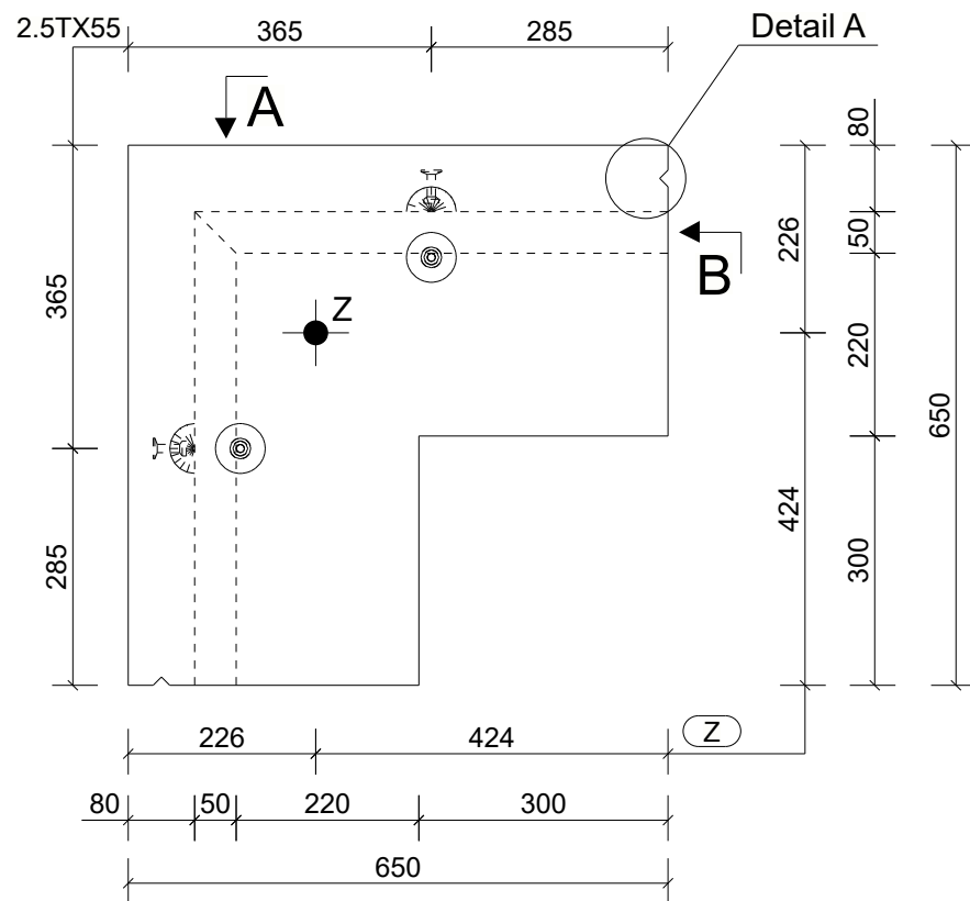
Aanzicht C Schaal: 1:10
