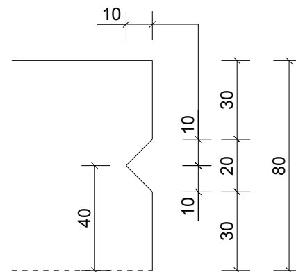
Detail A, 1:2
