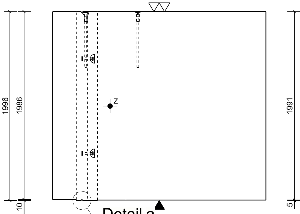
Aanzicht A Schaal: 1:25
