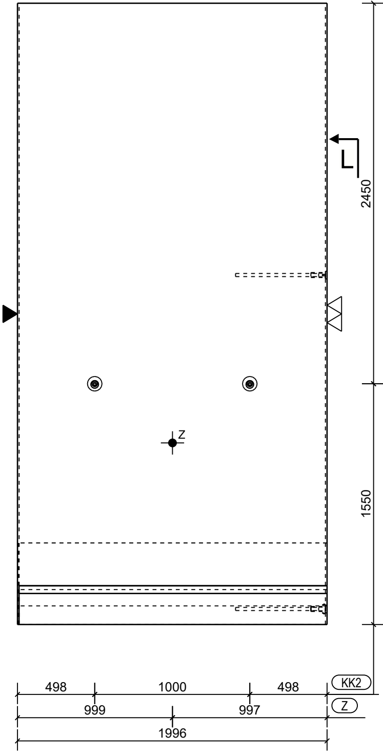
Aanzicht B Schaal: 1:25
