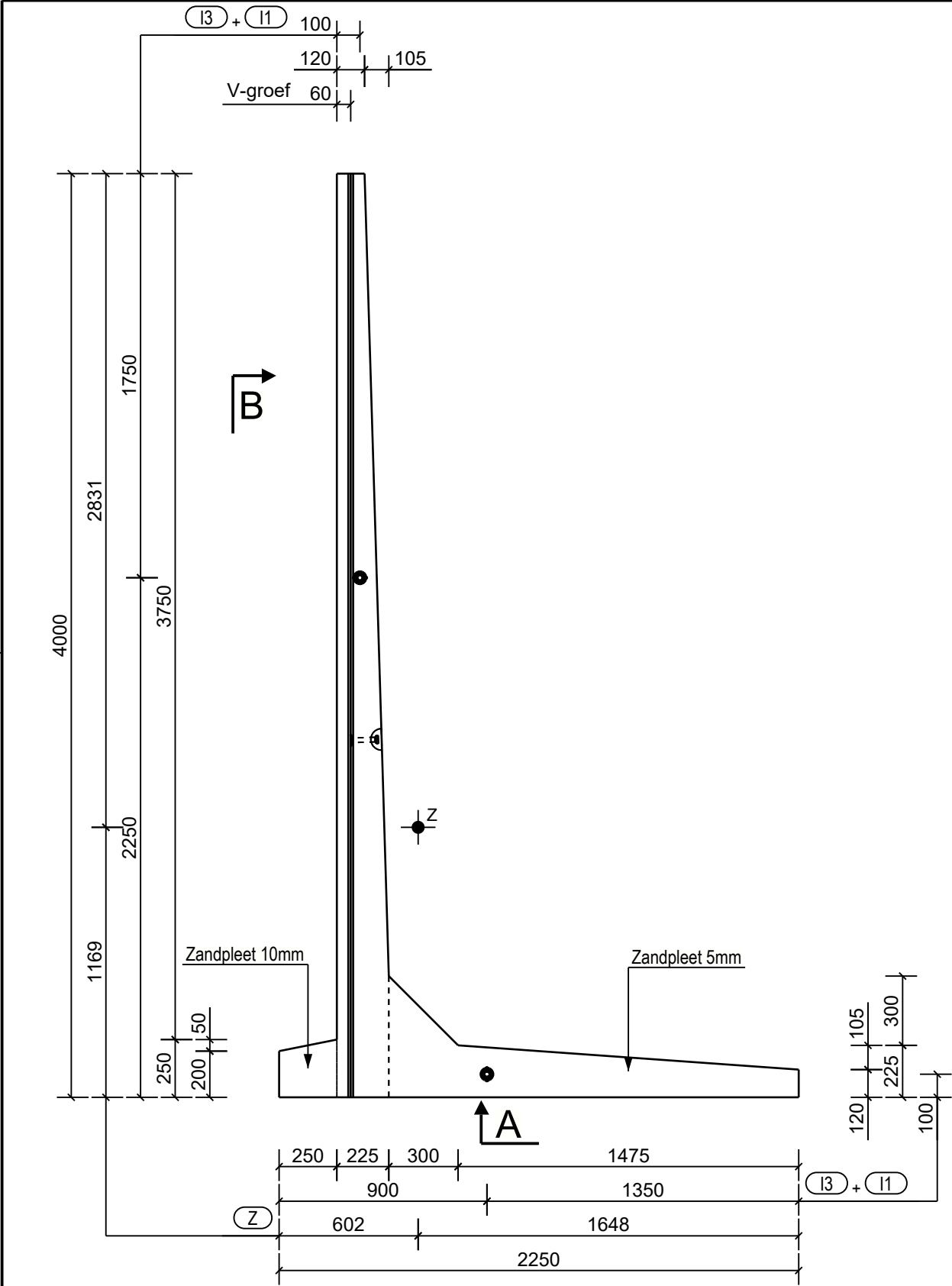
Zijaanzicht L (= aanzicht stortzijde) Schaal: 1:25
