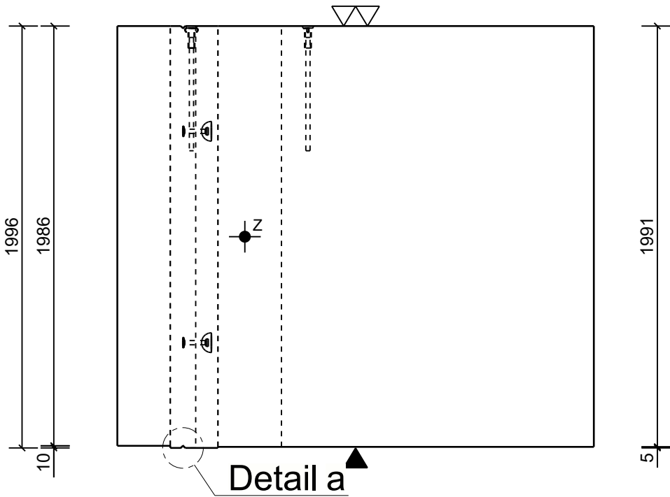
Aanzicht A Schaal: 1:25
