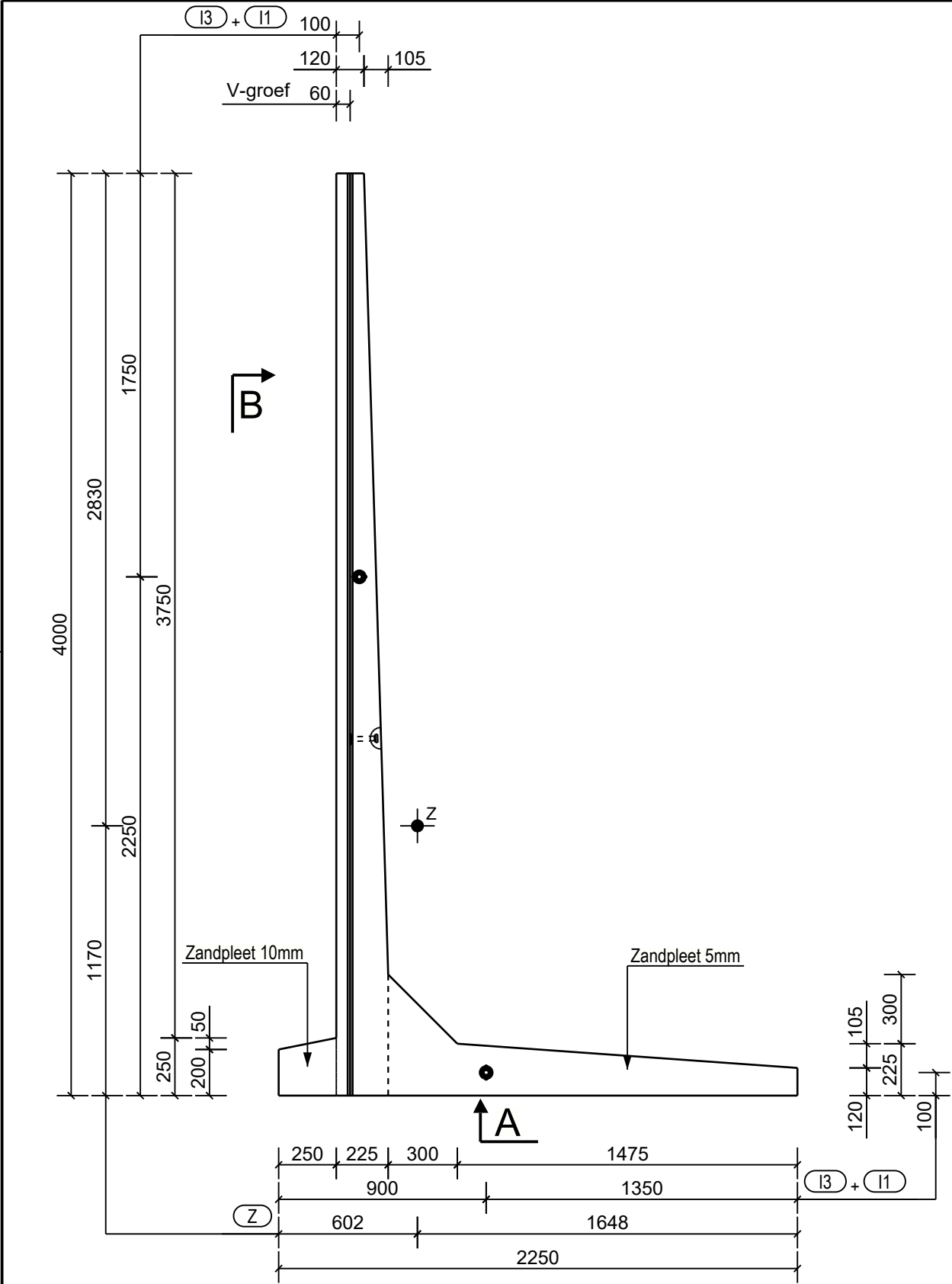
Zijaanzicht L (= aanzicht stortzijde) Schaal: 1:25
