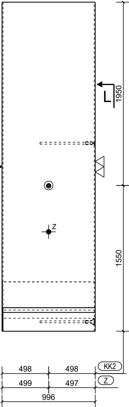
Aanzicht B Schaal: 1:25
