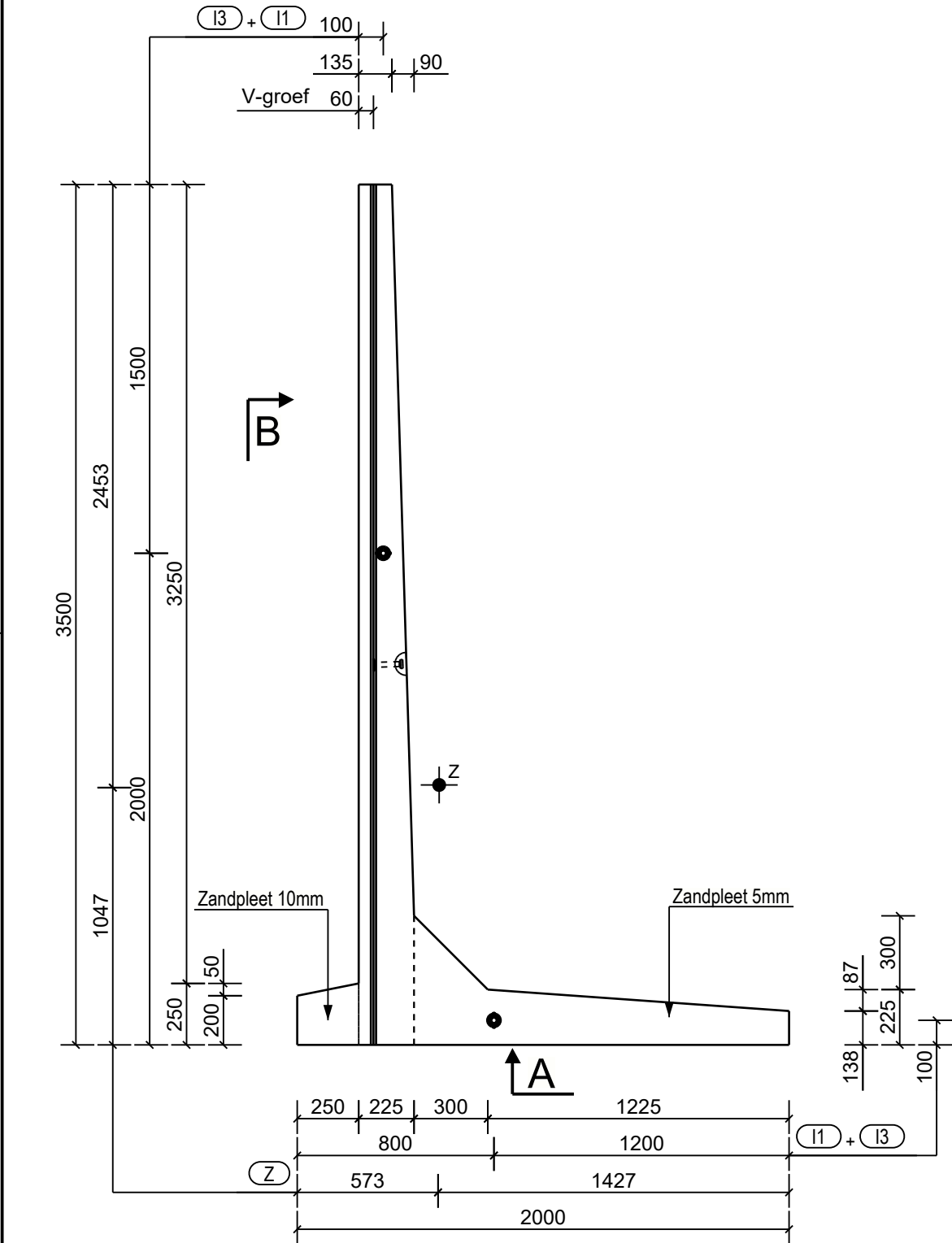
Zijaanzicht L (= aanzicht stortzijde) Schaal: 1:25
