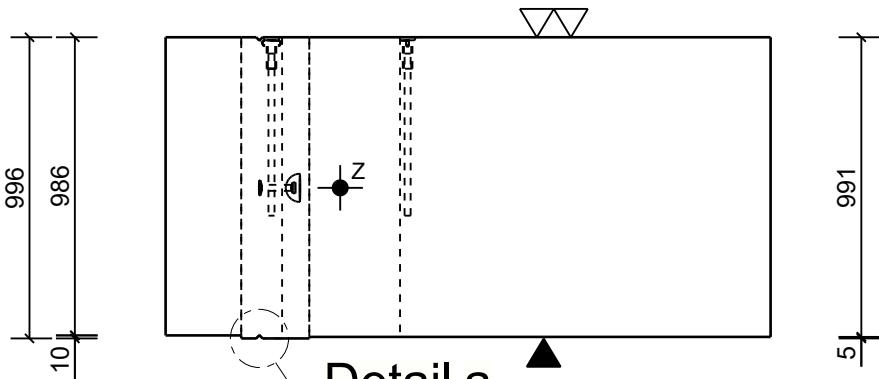
Aanzicht A Schaal: 1:25
