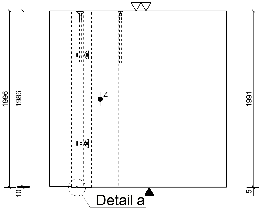
Aanzicht A Schaal: 1:25
