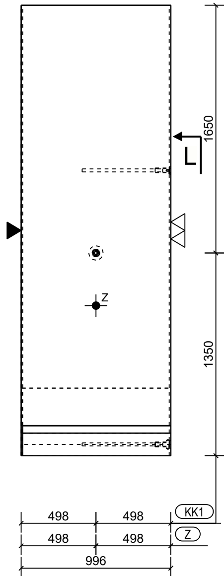
Aanzicht B Schaal: 1:25
