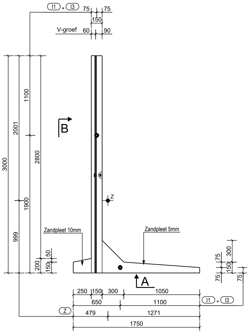
Zijaanzicht L (= aanzicht stortzijde) Schaal: 1:25
