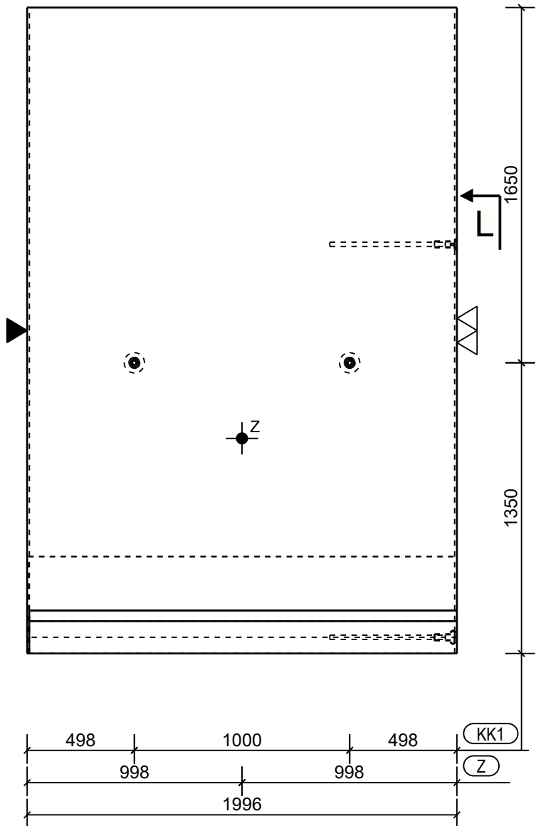
Aanzicht B Schaal: 1:25
