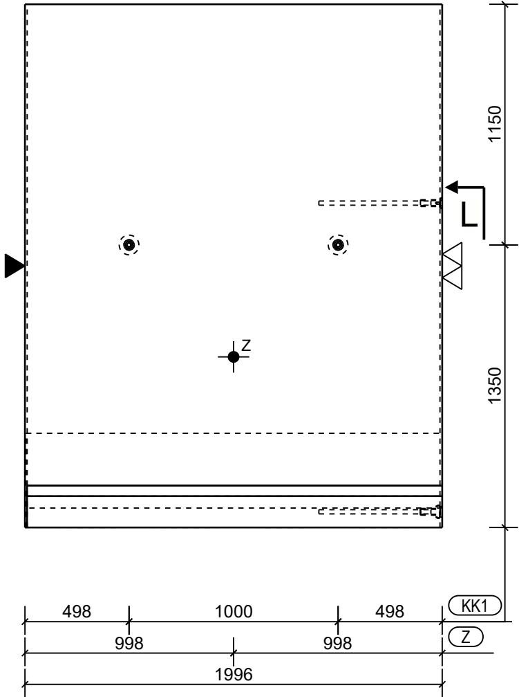
Aanzicht B Schaal: 1:25
