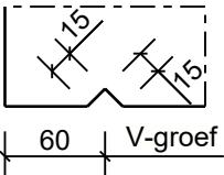
Detail a Schaal: 1:5
