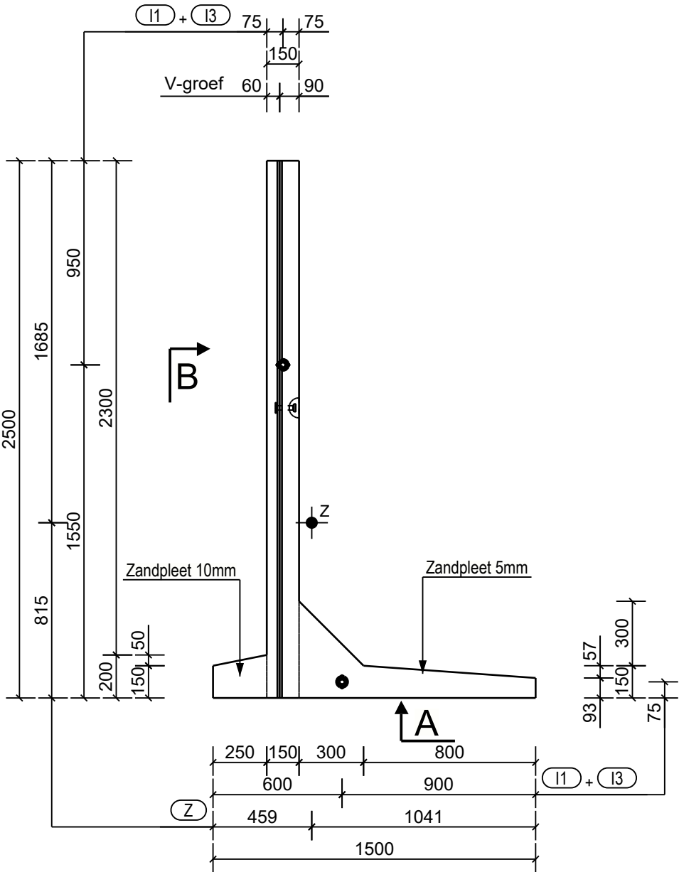
Zijaanzicht L (= aanzicht stortzijde) Schaal: 1:25
