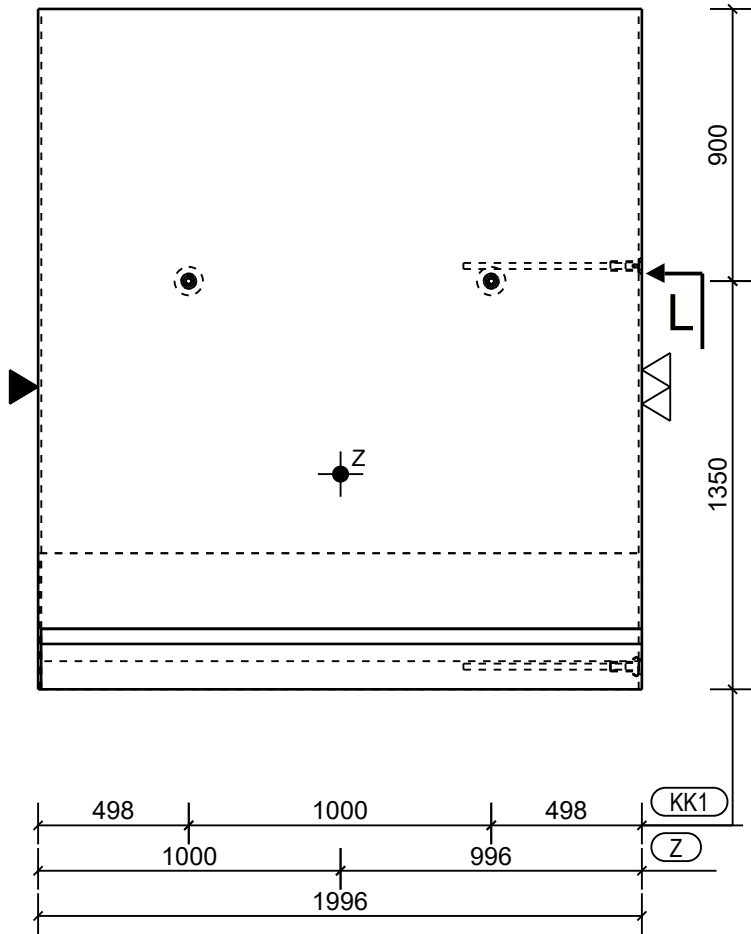
Aanzicht B Schaal: 1:25
