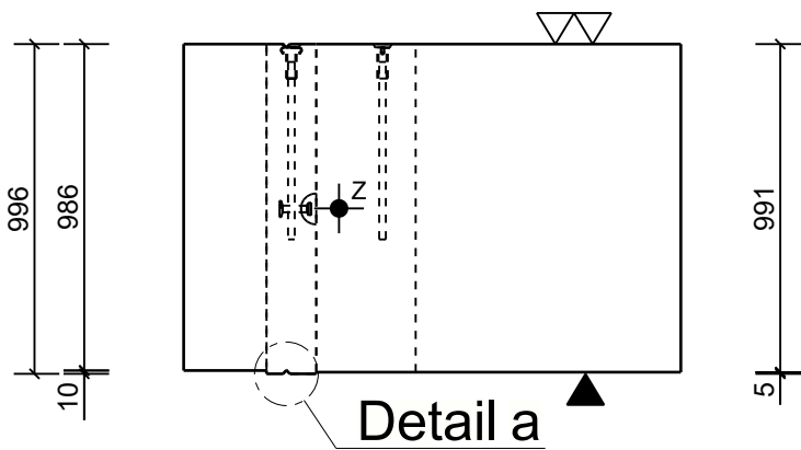
Aanzicht A Schaal: 1:25
