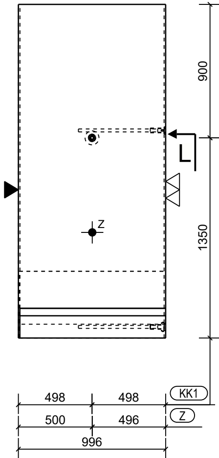
Aanzicht B Schaal: 1:25
