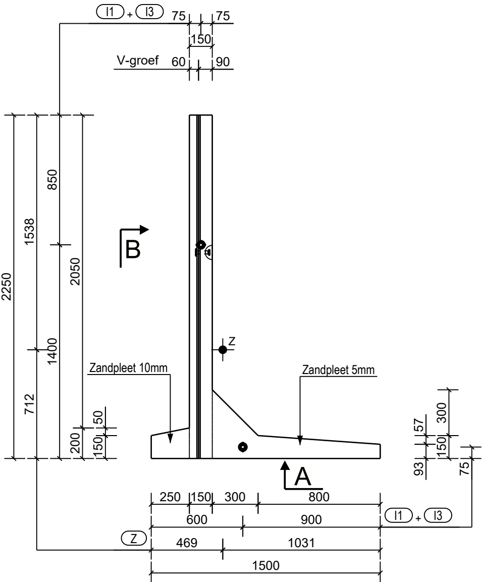
Zijaanzicht L (= aanzicht stortzijde) Schaal: 1:25
